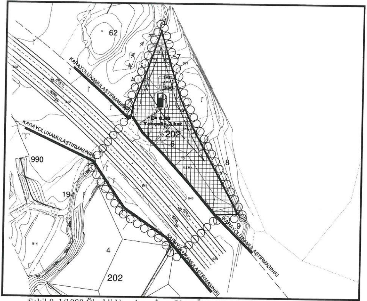
Şekil 8. 1/1000 Ölçekli Uygulama İmar Planı Örneği
