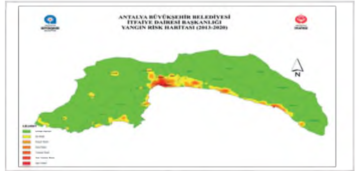
Resim: 2013-2020 Yılları Arasında Meydana Gelen Yangınlarına Göre Hazırlanan Yangın Risk Haritası
