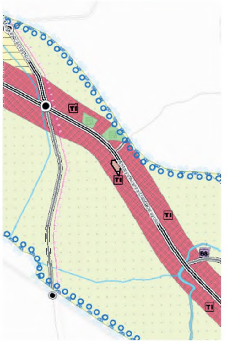
Resim: Manavgat İlçesi Doğançam Mahallesi Sınırları İçerisinde 1/25.000 ölçekli Nazım İmar Planı
