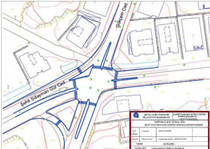
Resim: Şehit Süleyman Gür Caddesi ile Gökçeın Caddesi Kesişimi Geometrik Düzenleme Projesi
