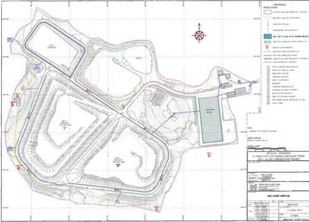
Şekil 3.9 Manavgat Katı Atık Düzenli Depolama ve Elektrik Üretim Tesisi genel vaziyet planı
