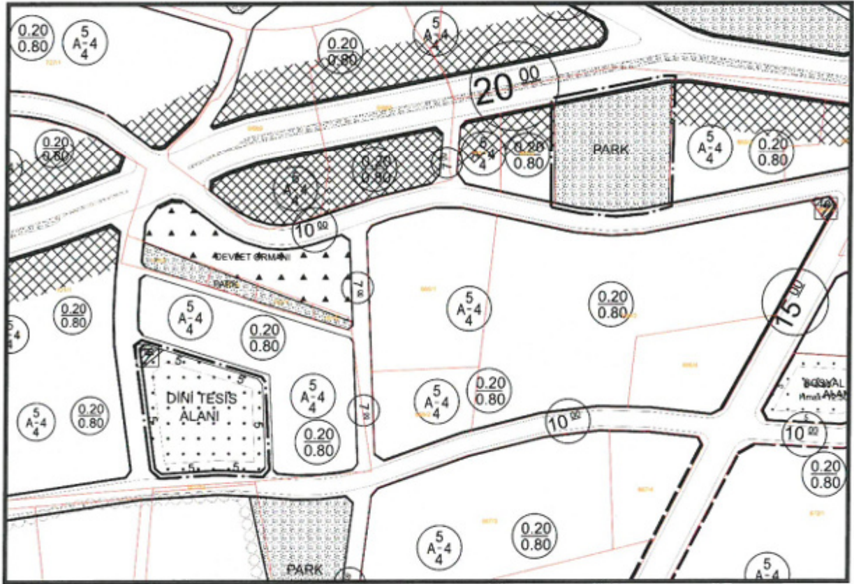
Şekil.5 Oba Mahallesi Meri 1/1000 Ölçekli Uygulama İmar Planı
