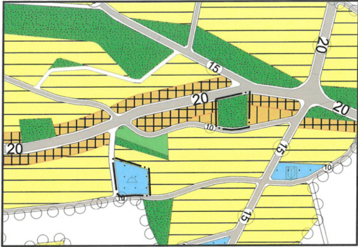
Şekil.3 Oba Mahallesi Meri 1/5000 Ölçekli Nazım İmar Planı
