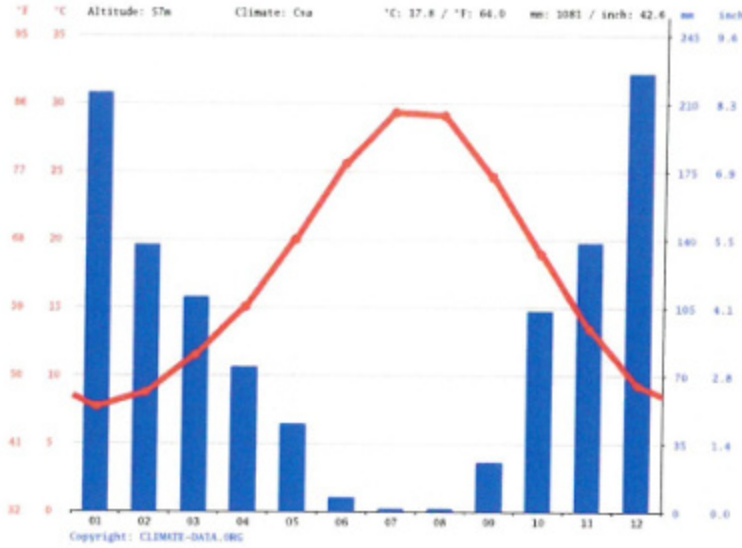
Şekil 1: İklim Grafiği
