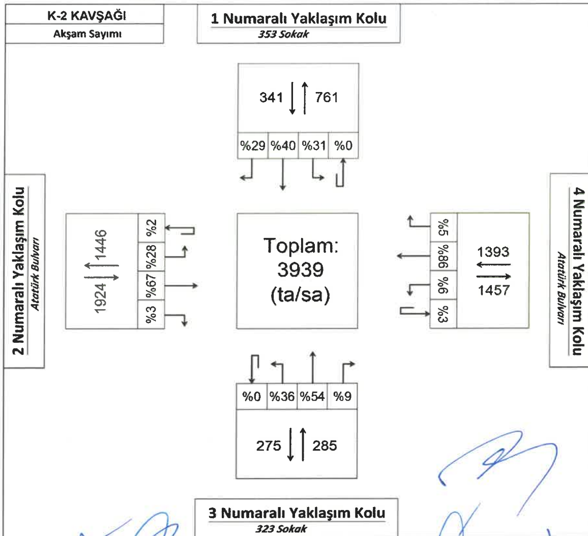
Şekil 28. K-2 kavşağı akşam sayımı saatlik trafik hacmi seması
