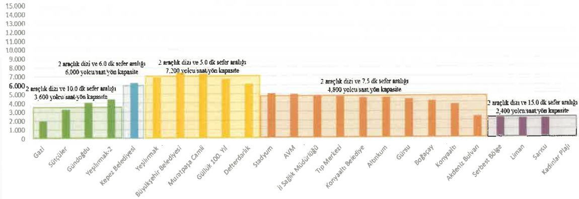
Şekil 137. 2025 Yılı Yolculuk Talebi - İşletme Sıklığı - Kapasite Grafiği
