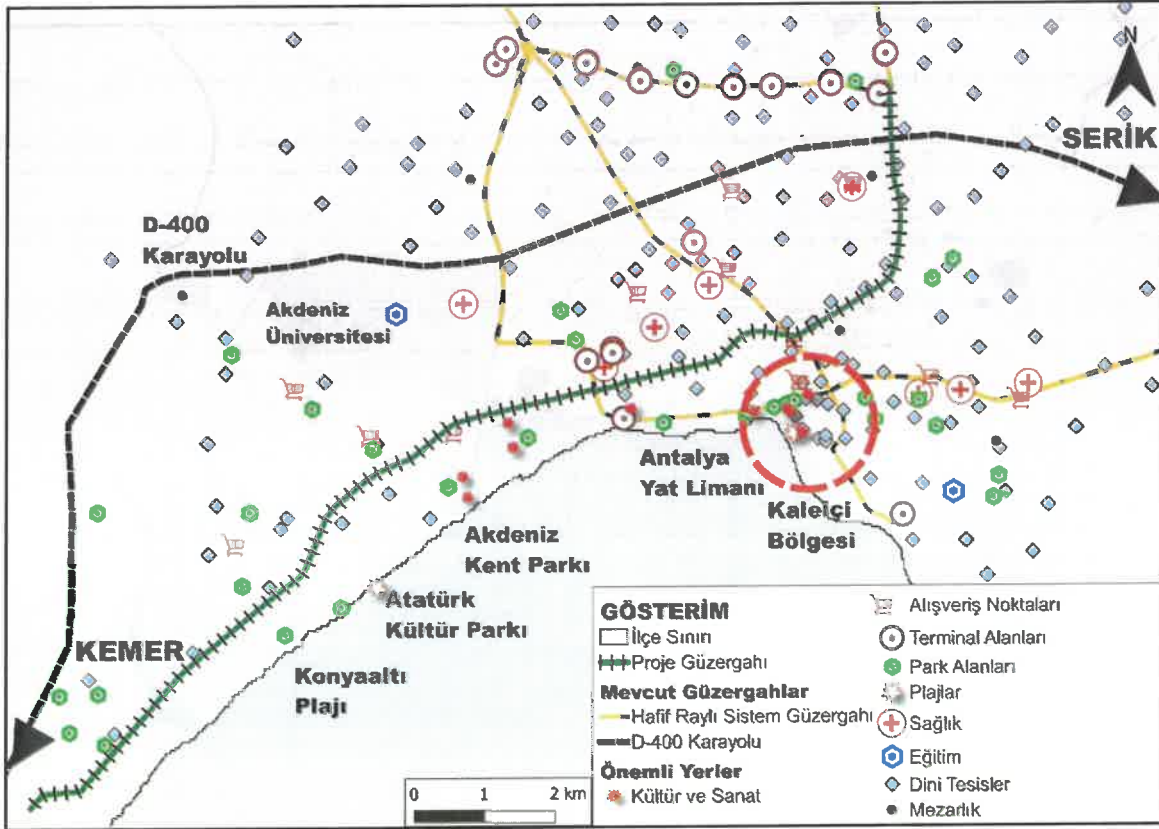
Şekil 101. Proje güzergahı yakın çevre analizi
