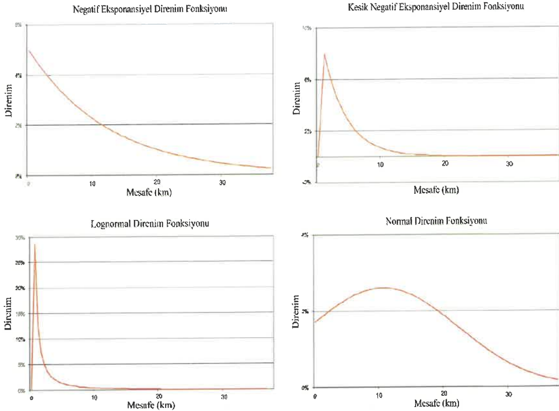
Şekil 108. Bazı direnir fonksiyonu yapıları (ICPSR, 2010)
