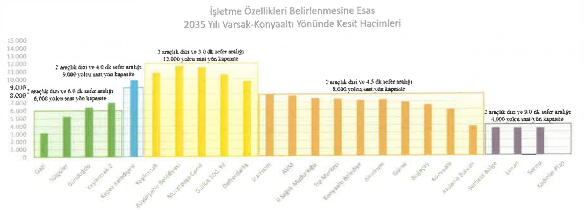
Şekil 139. 2035 Yılı Yolculuk Talebi - İşletme Sıklığı - Kapasite Grafiği
