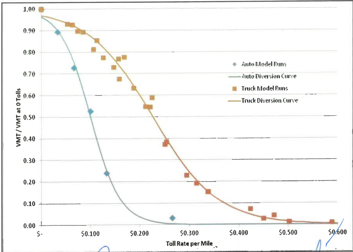
Şekil 117. Türlere göre sapma eğrisi (Erhardt & Brinckerhoff, 2013)
