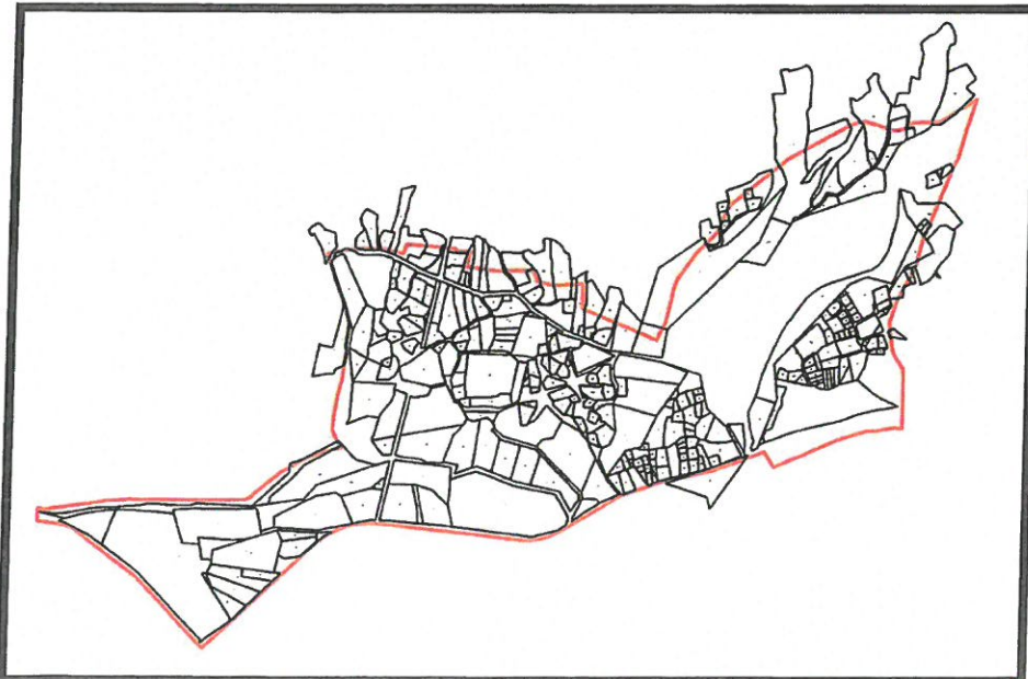
Şekil 2.Kadastral Durum
