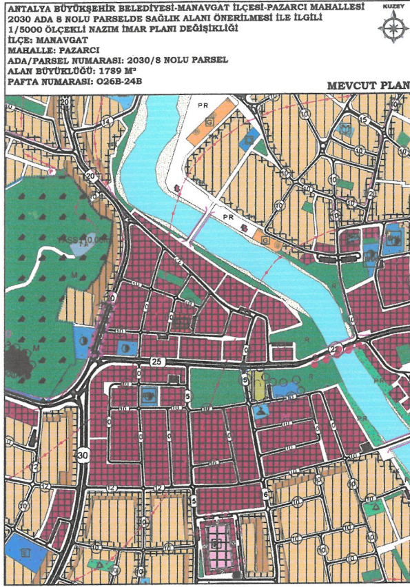
Şekil 4: Mevcut-Öneri 1/5000 Ölçekli Nazım İmar Planı Değişikliği
