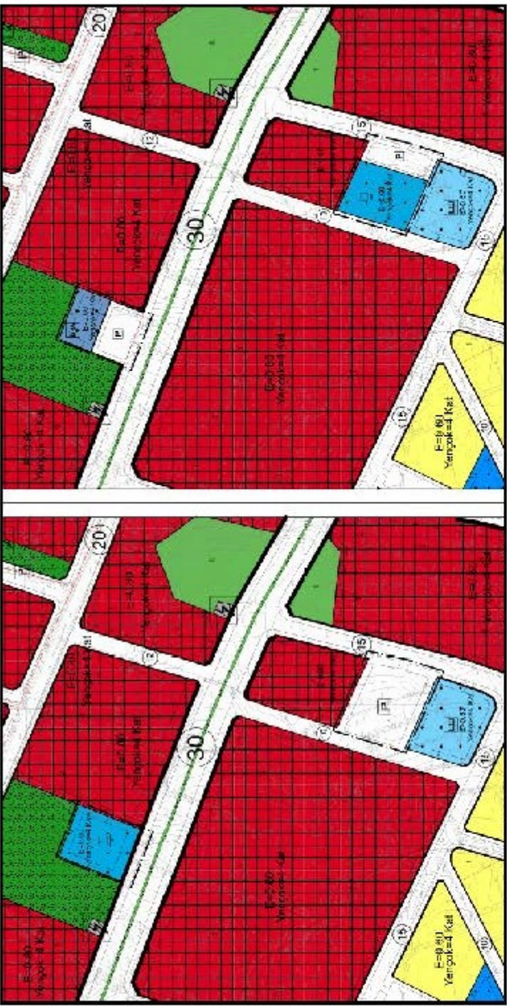
Plan 5: Mercut - Öneri 1/1000 Ölçekli Uygulama İmar Planı Değişikliği (Ölçeksiz)
