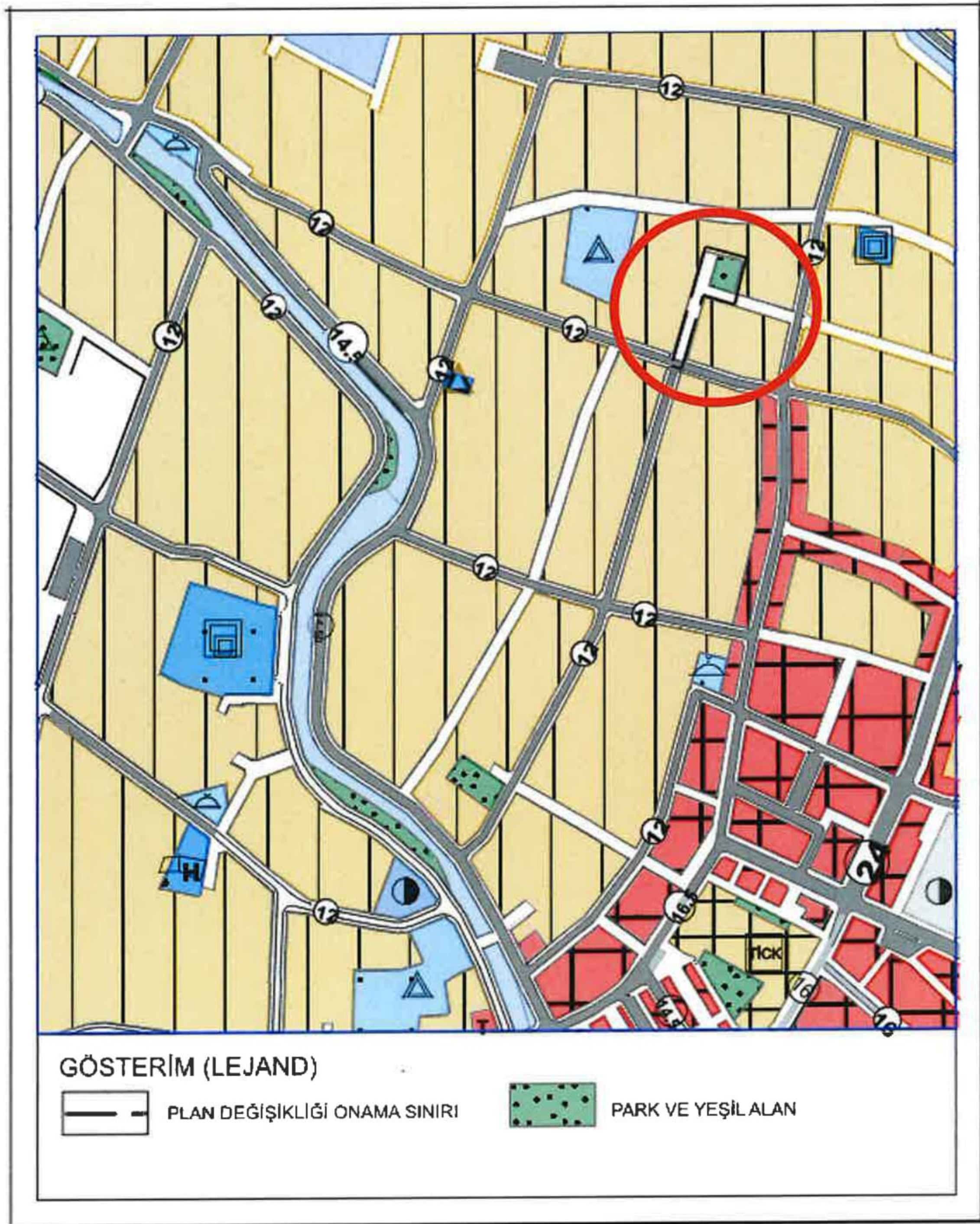
Plan 3: mevcut 1/5.000 Ölçekli Nazım İmar Planı (Ölçeksiz)
