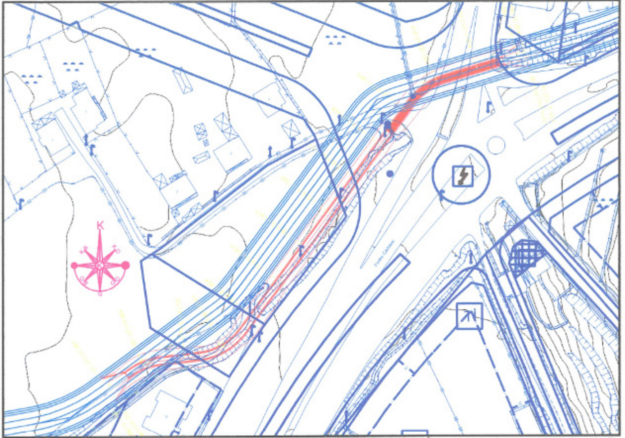
Proje 2: İmar Planı Üzerinde Çökelek Deresinin 28.10.2024 Tarih ve 5168519 Sayılı DSI 13. Bölge Müdürlüğü Yazısı Ekinde Revize Edilen Proje Güzergahı (Kırmızı Hat)
