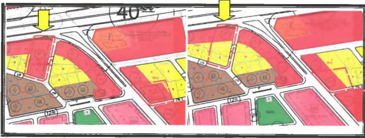
42. Mevcut ve Öneri 1/1000 Ölçekli Uygulama İmar Planı Değişikliği
