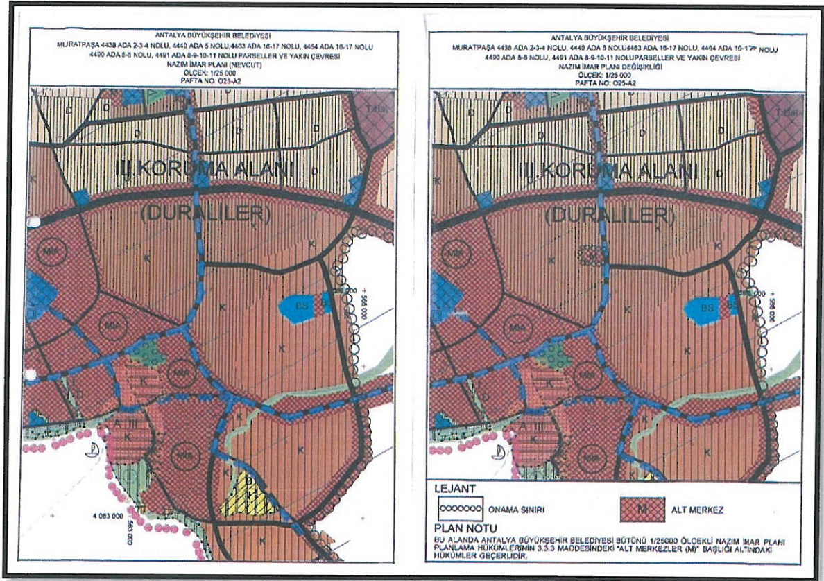
Şekil 11:13.11.2012/614 Sayılı Bbm(1/25000 Ölçekli Nazım İmar Planı).
