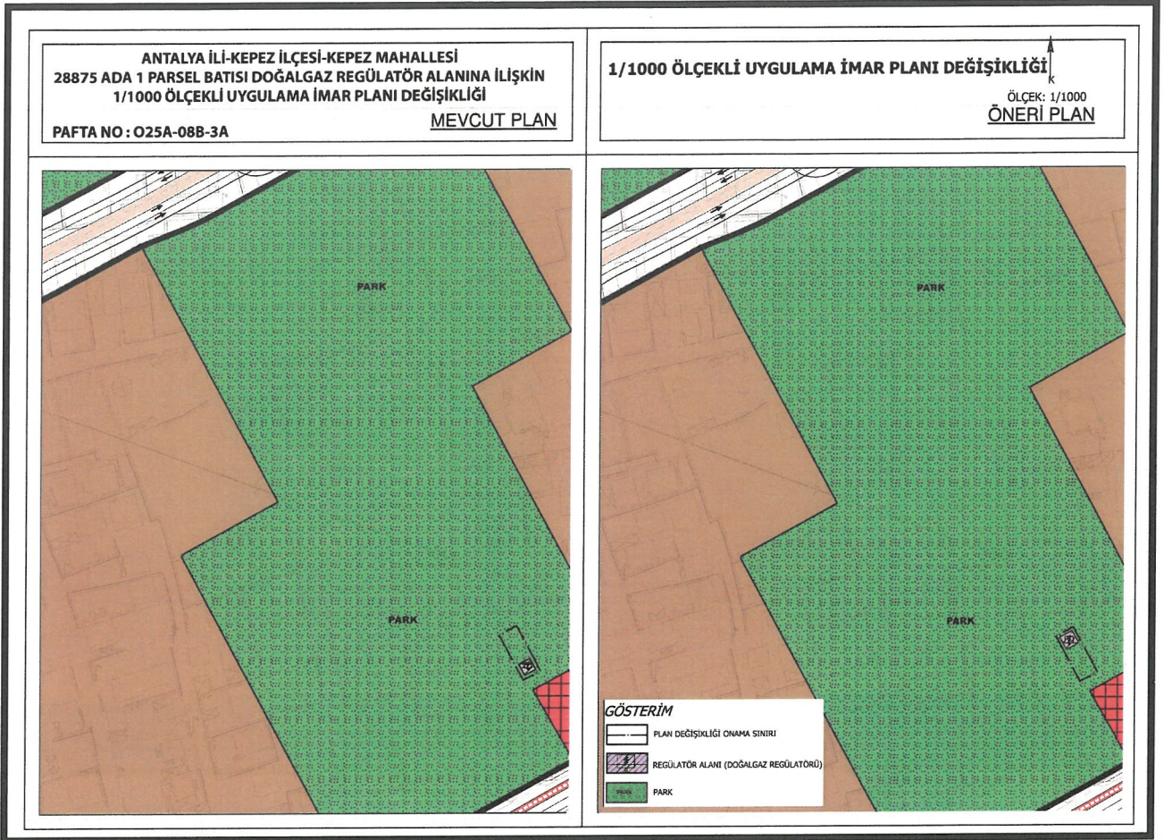
Şekil 7. 1/1000 ölçekli Uygulama İmar Planı Örneği
